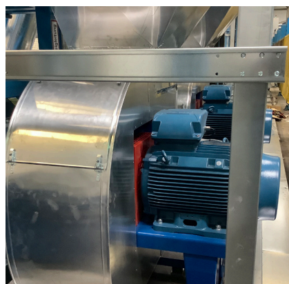
Ventilator mit schalldämmender Isolierung
